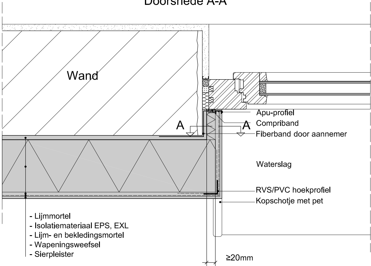
Doorsnede A-A
