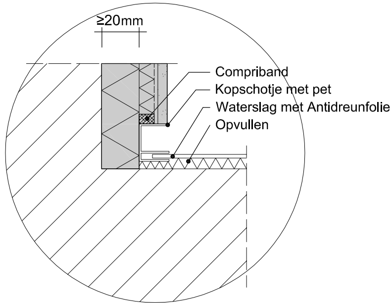
Doorsnede A-A
