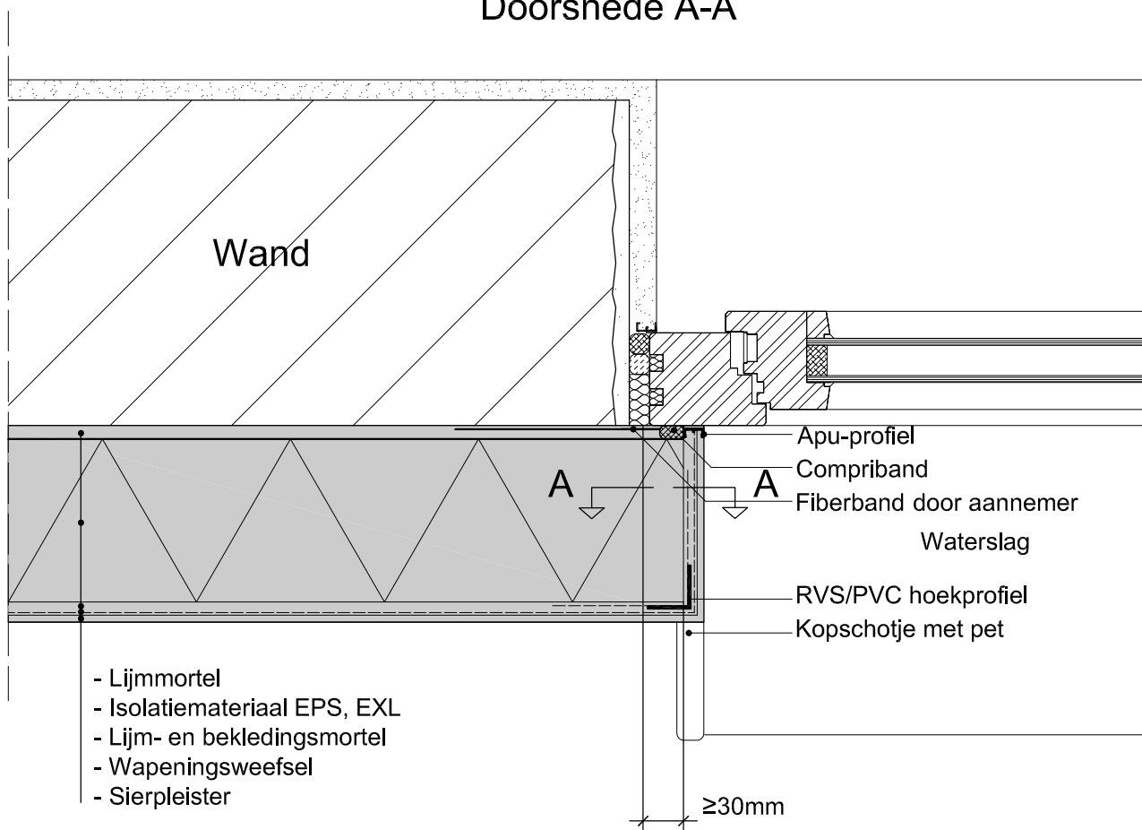
Doorsnede A-A
