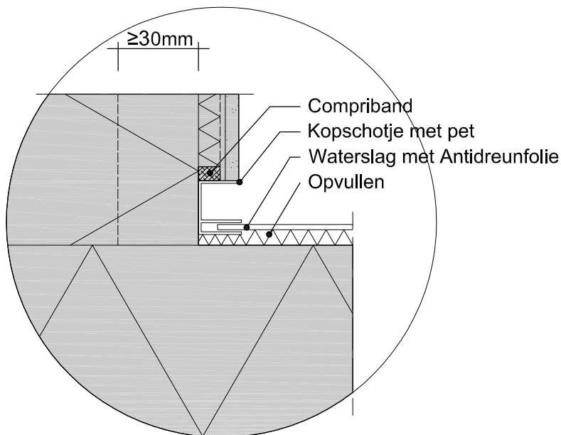
Doorsnede A-A
